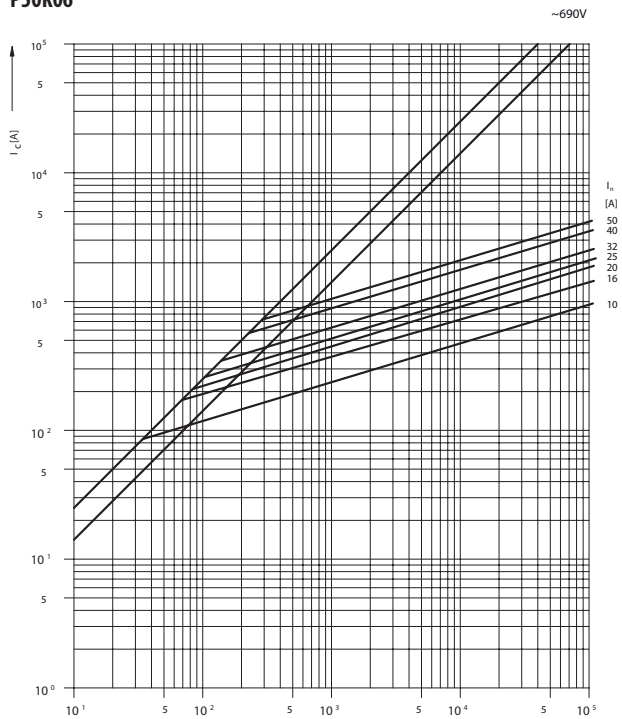
Omezovací charakteristika P50K06
